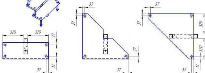
Схема расположения ступеней относительно элементов каркаса модульной лестницы и разметка для засверливания под болты крепления балки и стоек перил (отверстие \varnothing 9 мм) и прямоугольных сквозных отверстий под стойки (отверстие \varnothing 26 мм)
