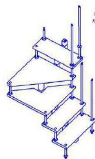
Схема расположения ступеней относительно элементов каркаса модульной лестницы и разметка для засверливания под болты крепления балки и стоек перил (отверстие \varnothing 9 мм) и прямоугольных сквозных отверстий под стойки (отверстие \varnothing 26 мм)
